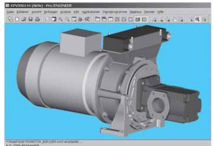
Kühlpumpenträger Serie KPV mit Fußflansch PTFL Cooler-bellhousing series KPV with footflange PTFL
